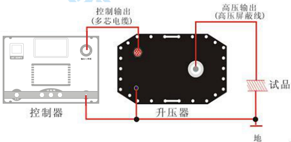
图 4 (连线图)
