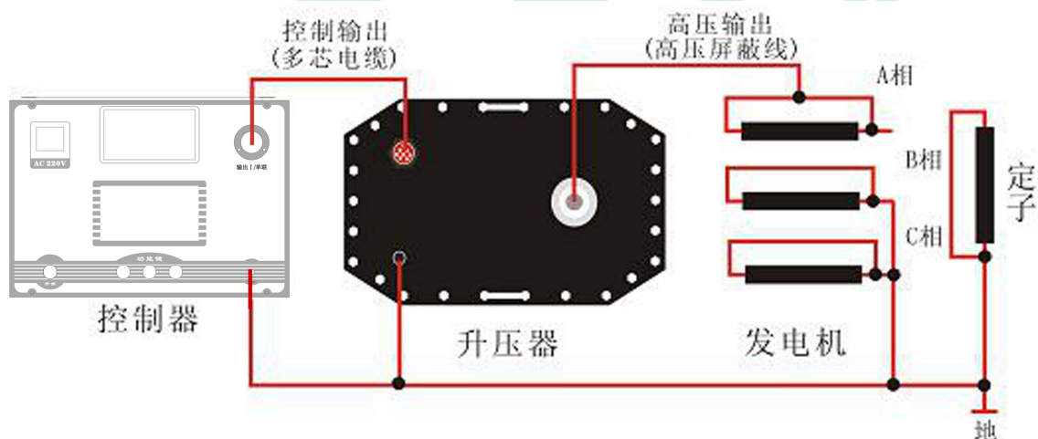
图 14 测量定子的某相连线图
