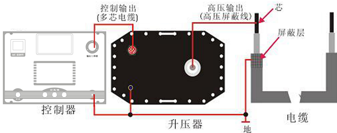
图 13 单相测量连线图
