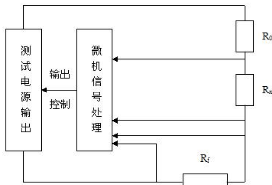
图 1 测量原理示意图
