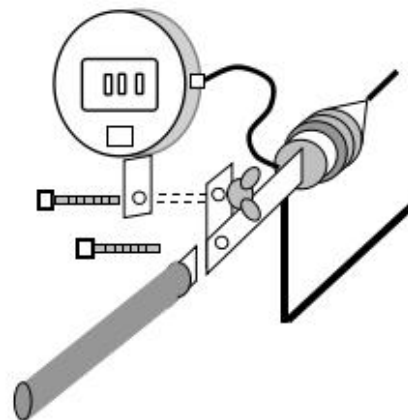
装配图
