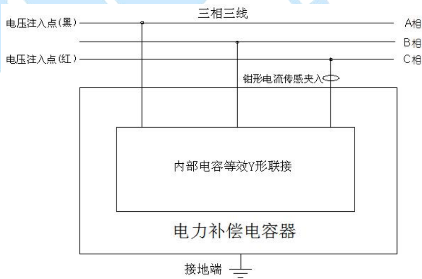
图 27 Y 形联接被试电容 CA 相接线图
