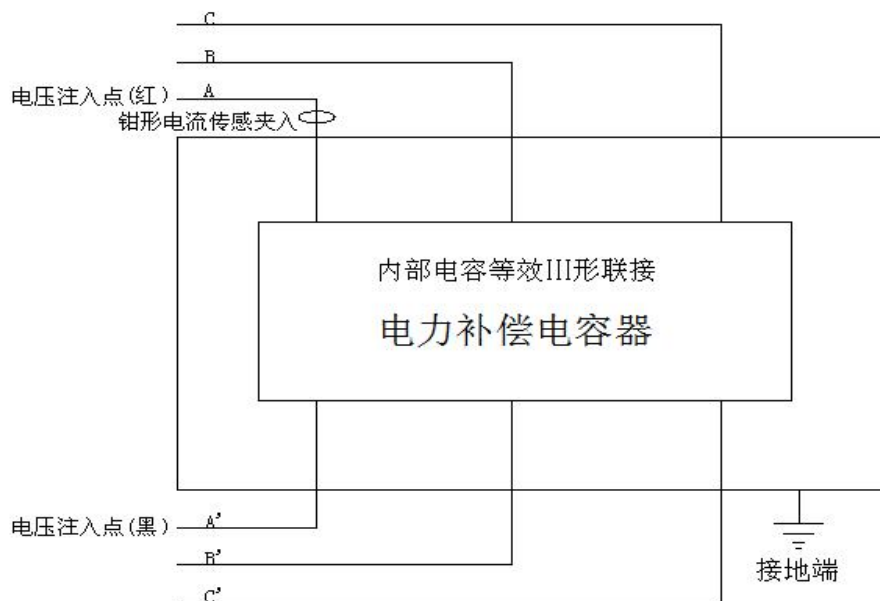
图 31 III形联接被试电容接线图
