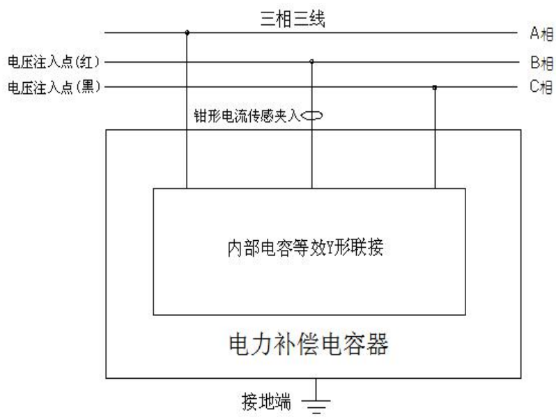
图 26 Y 形联接被试电容 BC 相接线图
