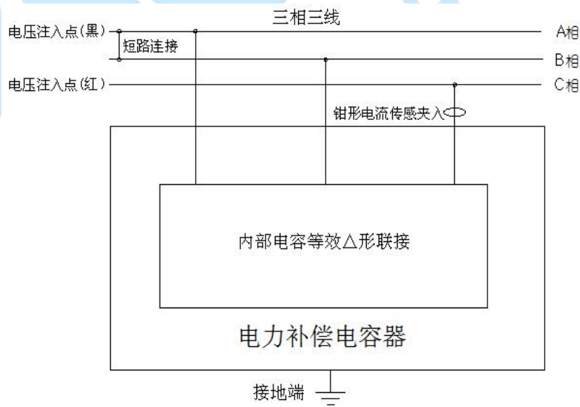
图 24 \Delta 形联接被试电容 CA 相接线图
