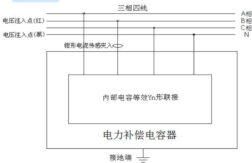
图 29 Yn 形联接被试电容 Bn 相接线图
