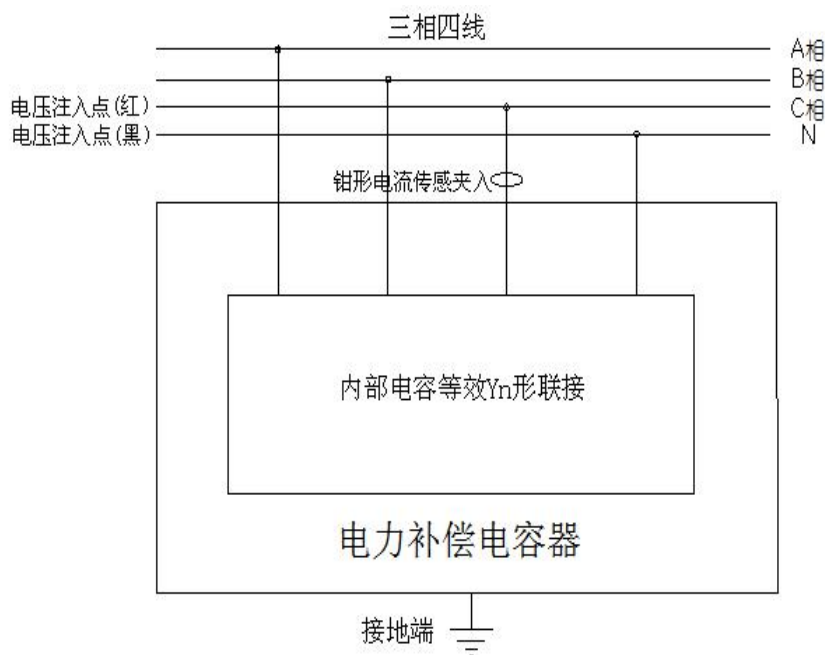
图 30 Y_n 形联接被试电容 C_n 相接线图
