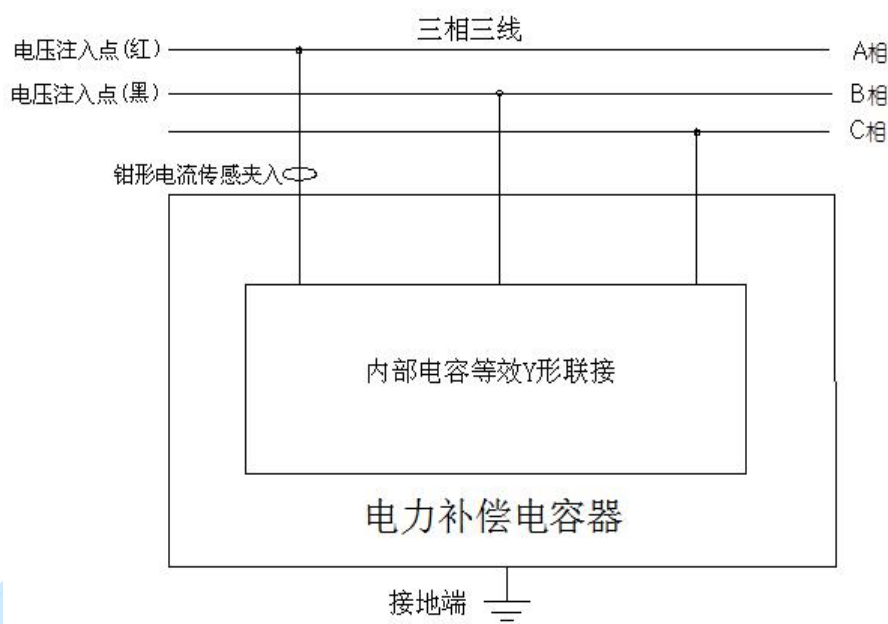
图 25 Y 形联接被试电容 AB 相接线图
