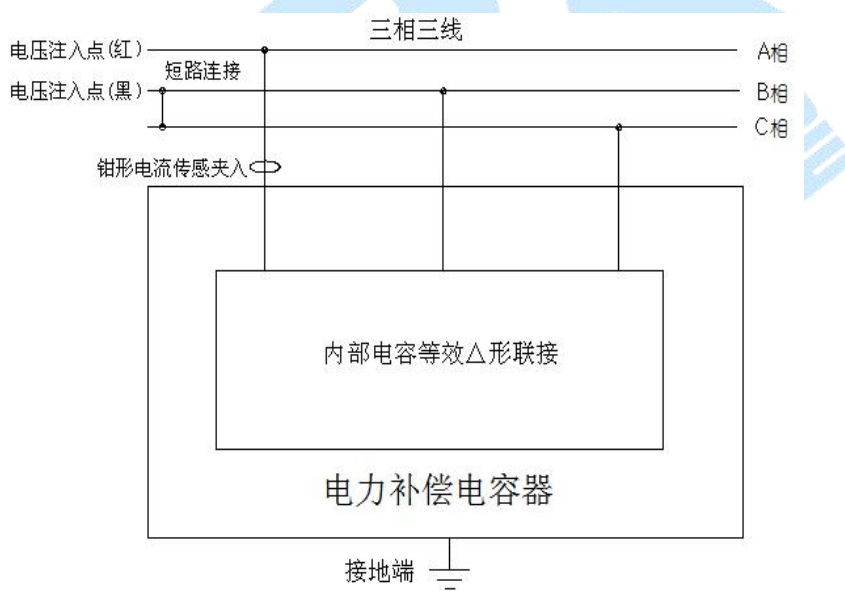
图 22 \Delta 形联接被试电容 AB 相接线图
