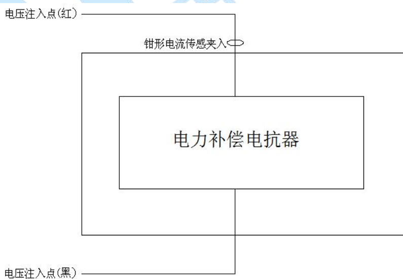
图 32 被试电抗器电感接线图
