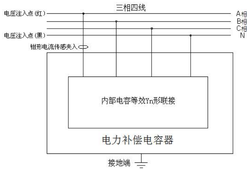
图 28 Yn 形联接被试电容 An 相接线图
