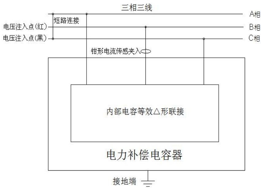
图 23 \Delta 形联接被试电容 BC 相接线图
