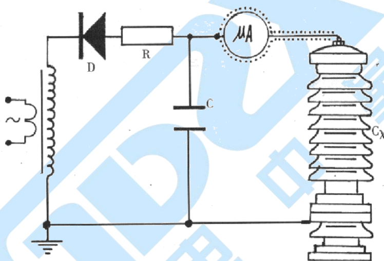
微安表接入试品 CX 高压侧接线图
