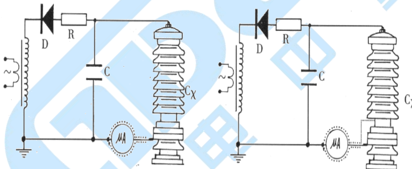
图 8a 微安表接入试品 C_x 底部的接线图
